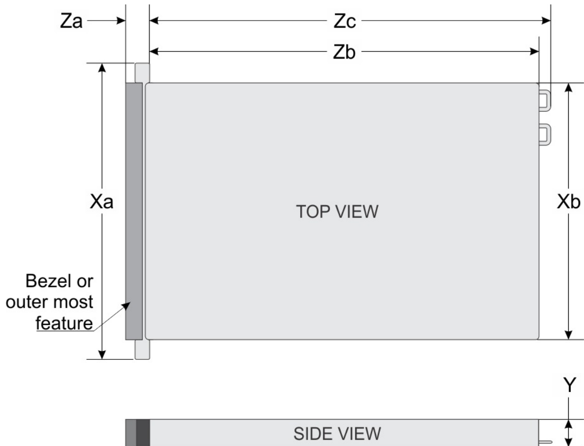
图 18: PowerEdge R450 机箱尺寸
