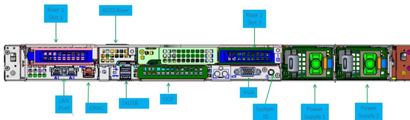
图 3: 系统的后视图
